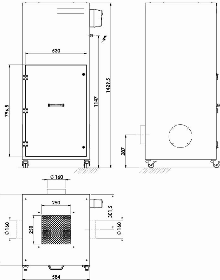
Dimensions du dépoussiéreur
